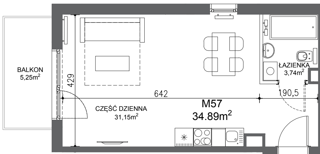
RZUT MIESZKANIA
