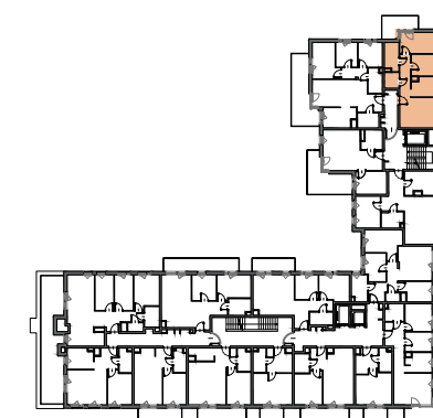
SCHEMAT KONDYGNACJI
