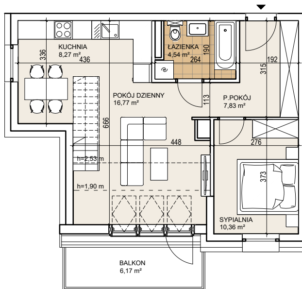
Poziom 1
