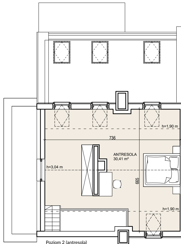
Poziom 2 (antresola)
