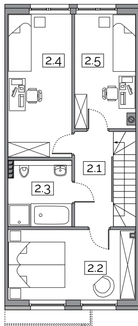
Piętro 54,24 m 2
