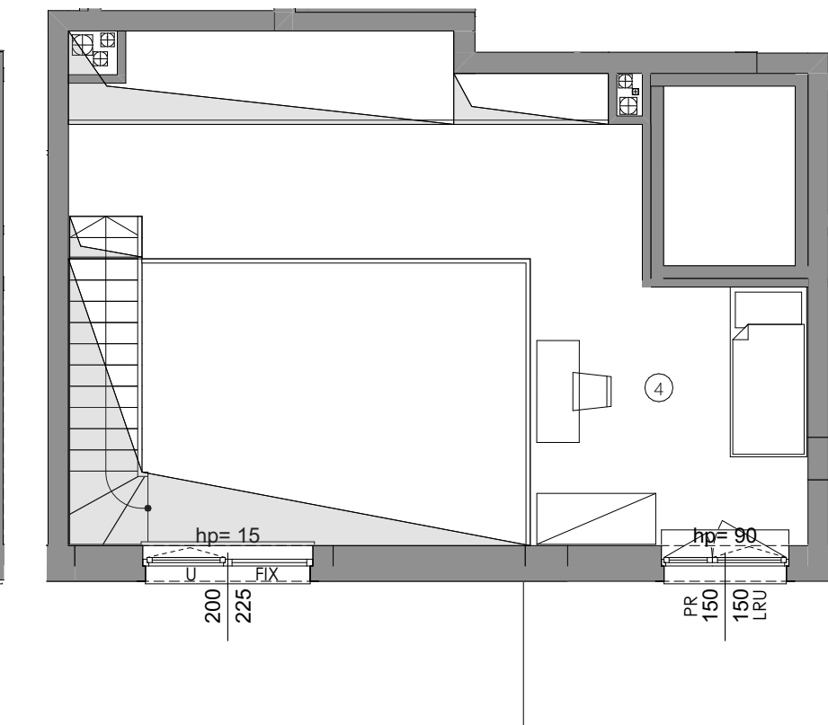
POZIOM ANTRESOLI
