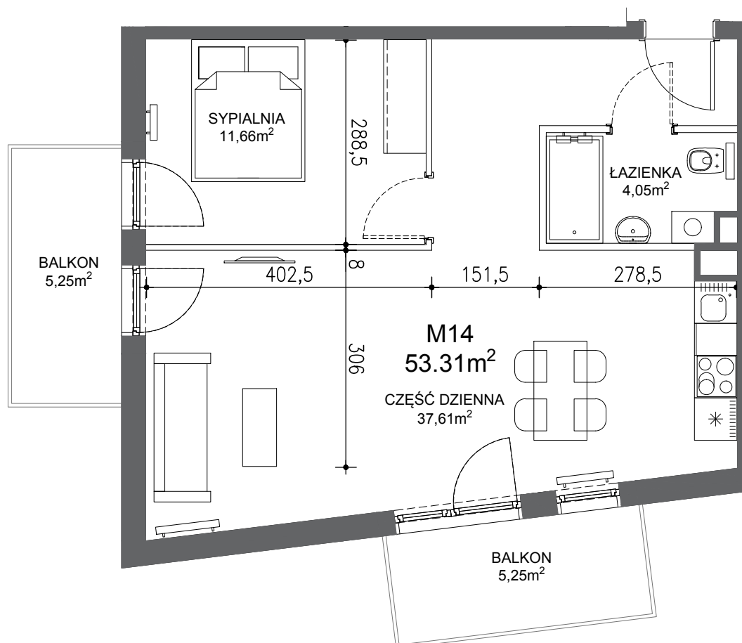
RZUT MIESZKANIA
