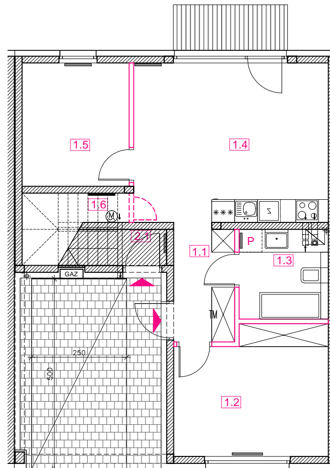
RZUT PARTERU
