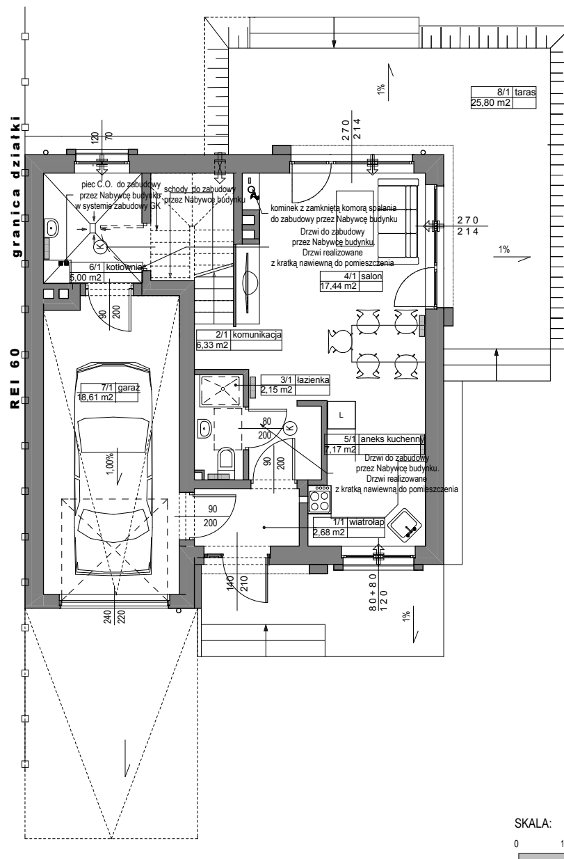
VILLA CAMPINA OŻARÓW MAZOWIECKI, SZEREG F06 - BUDYNEK ALICJA SKRAJNY O SZER.910cm., MODUŁ S128
