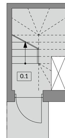
RZUT PARTERU
