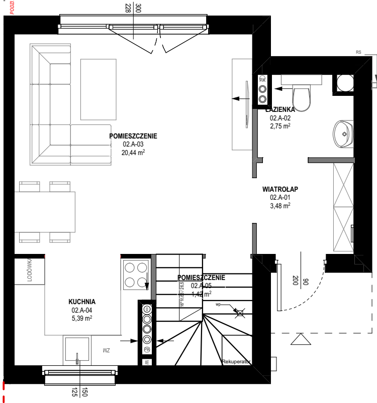
RZUT PARTERU
