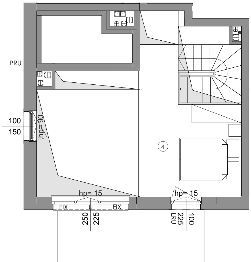
POZIOM ANTRESOLI
