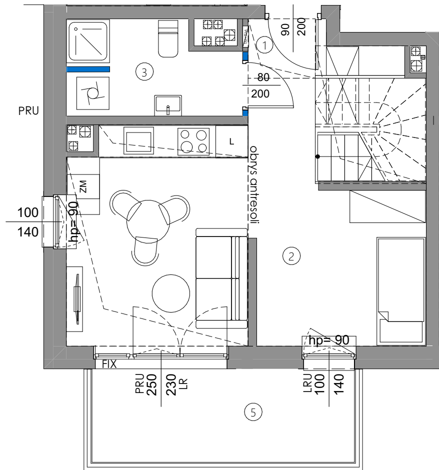
POZIOM DOLNY
