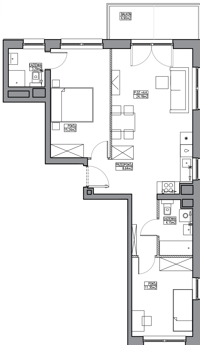
SCHEMAT LOKALU MIESZKALNEGO NA 1 PIĘTRZE
