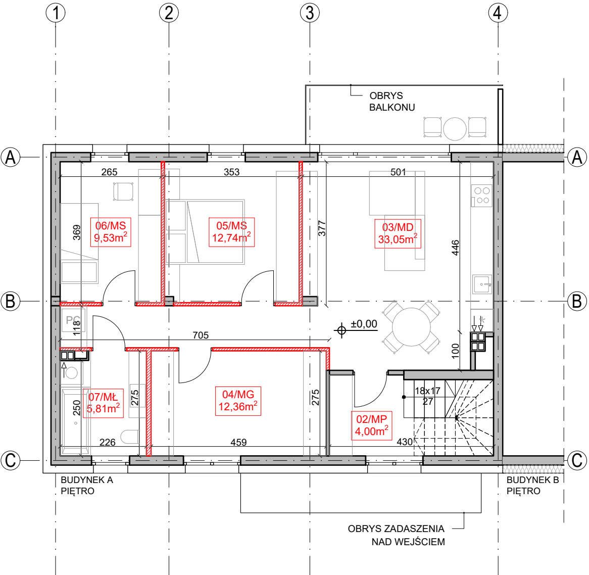
RZUT PIĘTRA
