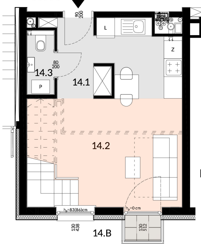
POZIOM 0
