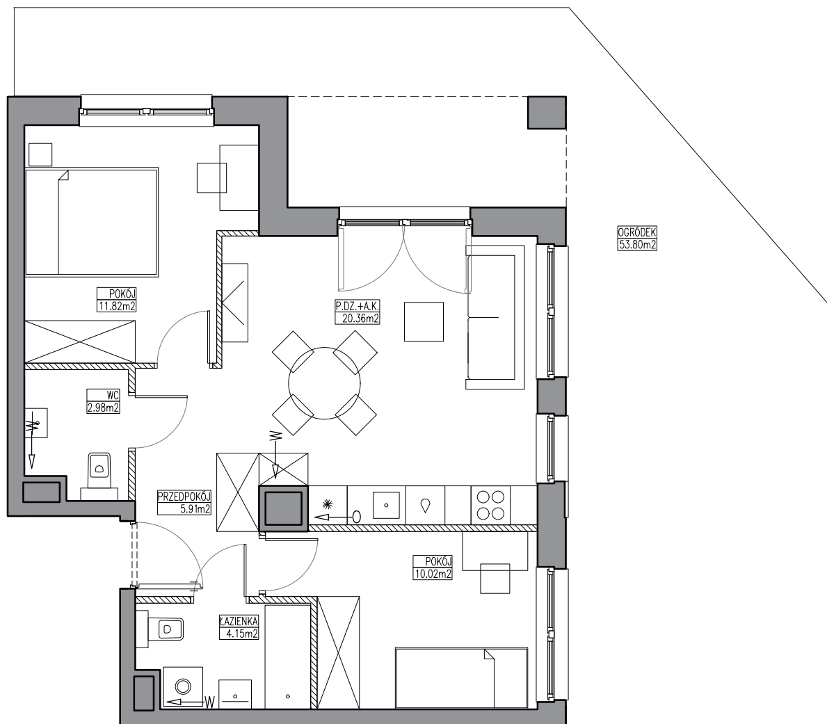
SCHEMAT LOKALU MIESZKALNEGO NA PARTERZE
