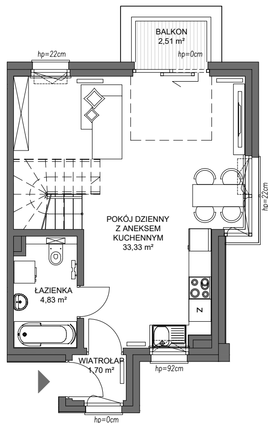
POZIOM 1
