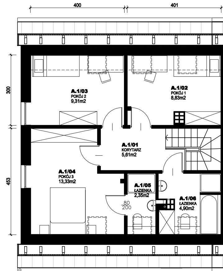
RZUT PODDASZA
