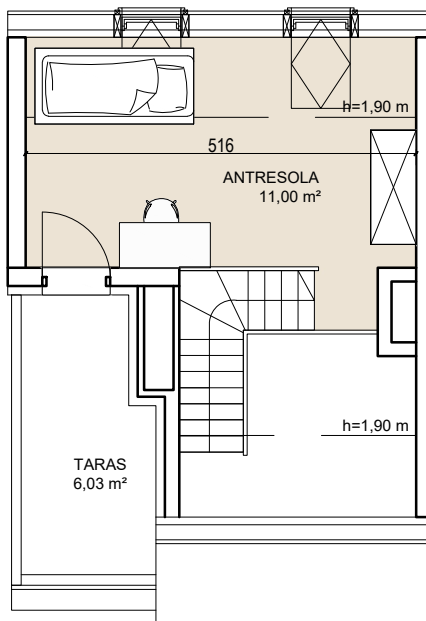
Poziom 2 (antresola)
