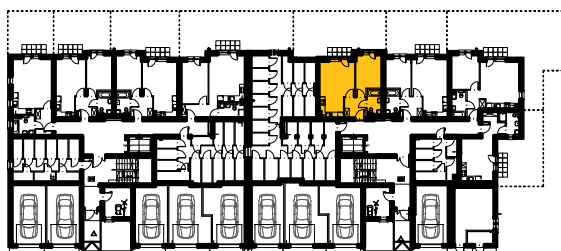
RZUT PARTERU
