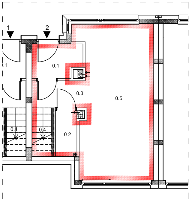
RZUT PARTERU BUDYNKU NR 9H LOKAL MIESZKALNY NR 2
