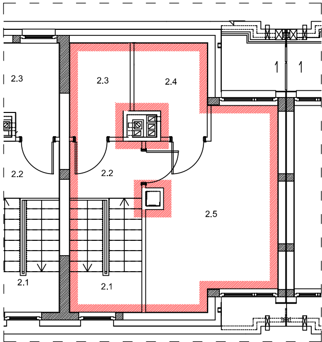
RZUT PIĘTRA II-GO BUDYNKU NR 9H LOKAL MIESZKALNY NR 2
