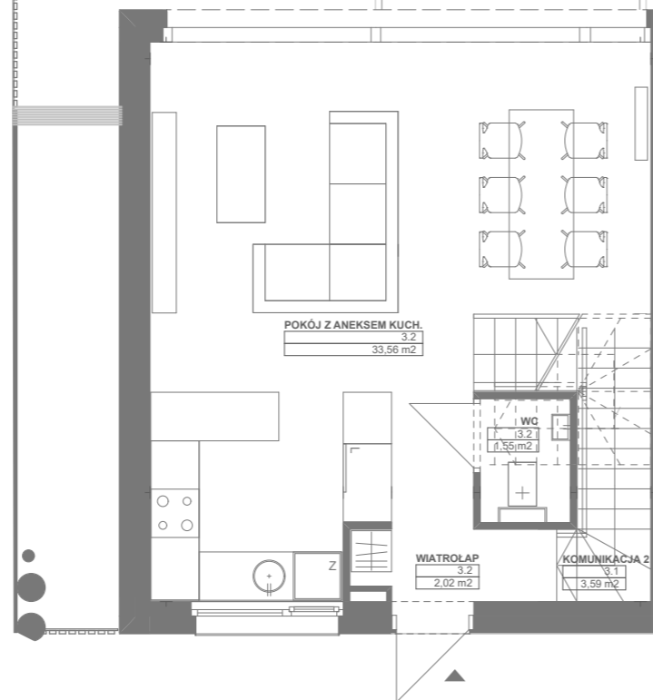
RZUT PARTERU
