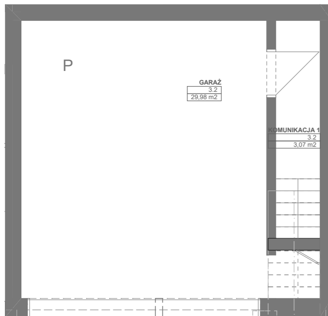
RZUT GARAŻU
