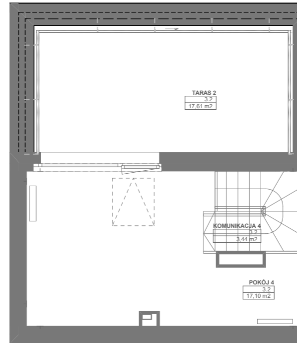
RZUT II PIĘTRA
