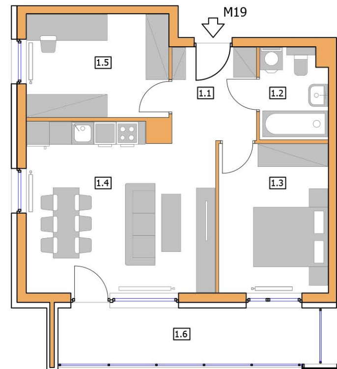
RZUT 1:100
