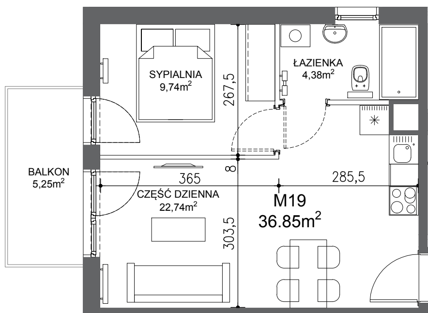
RZUT MIESZKANIA
