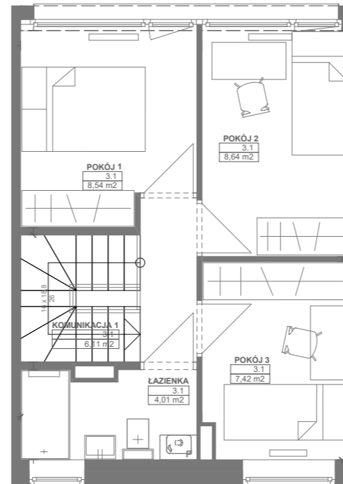
RZUT I PIĘTRA
