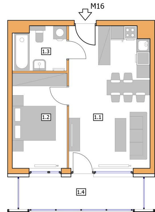
RZUT 1:100
