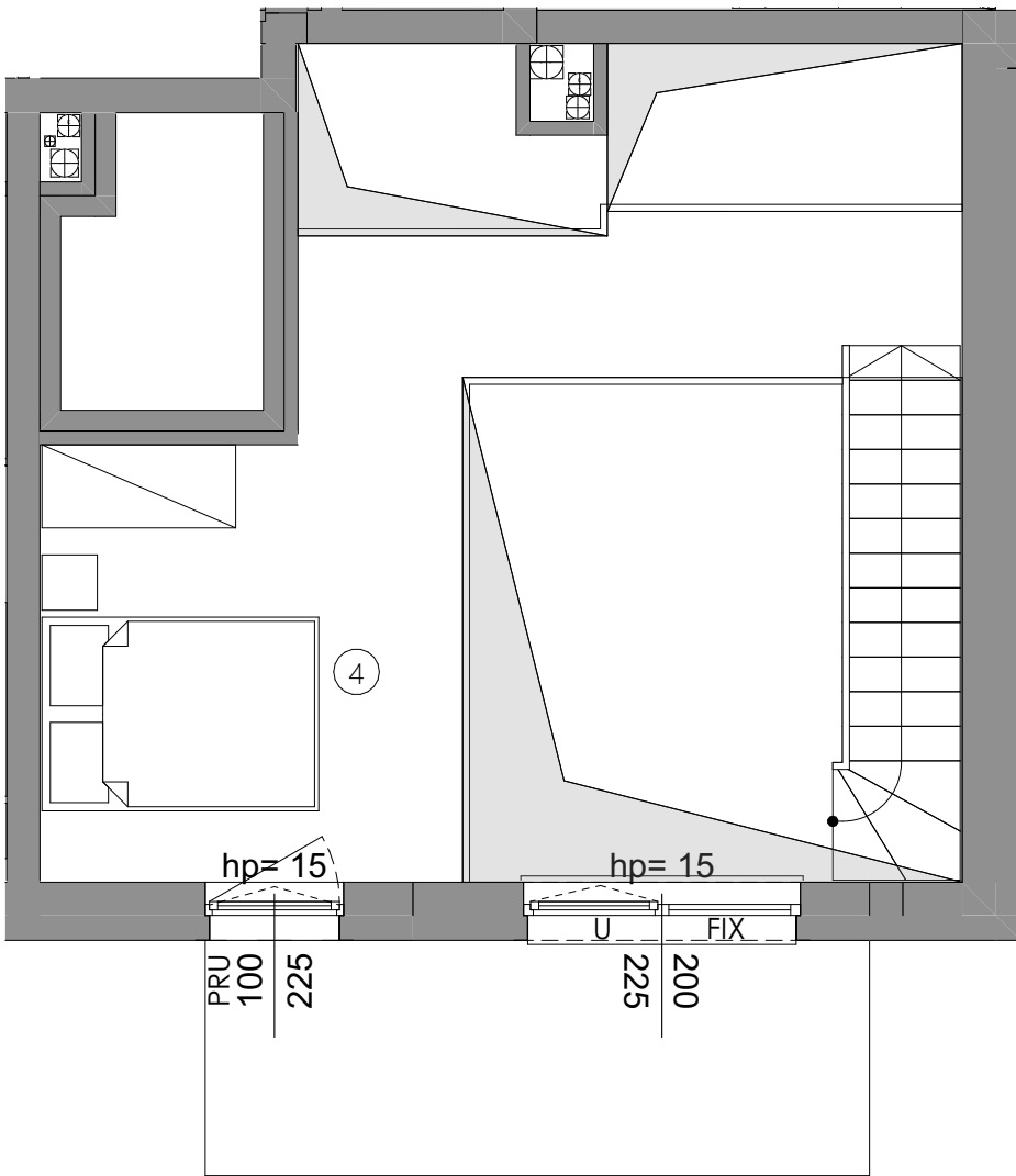
POZIOM ANTRESOLI
