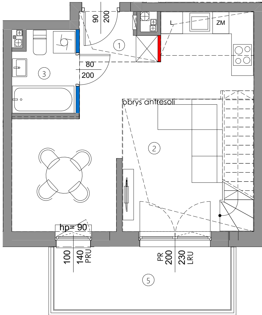
POZIOM DOLNY
