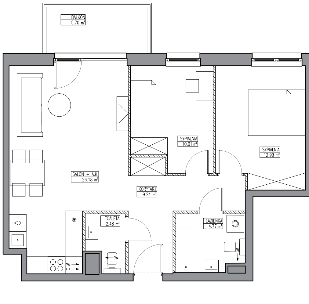
SCHEMAT LOKALU MIESZKALNEGO NA 7 PIĘTRZE
