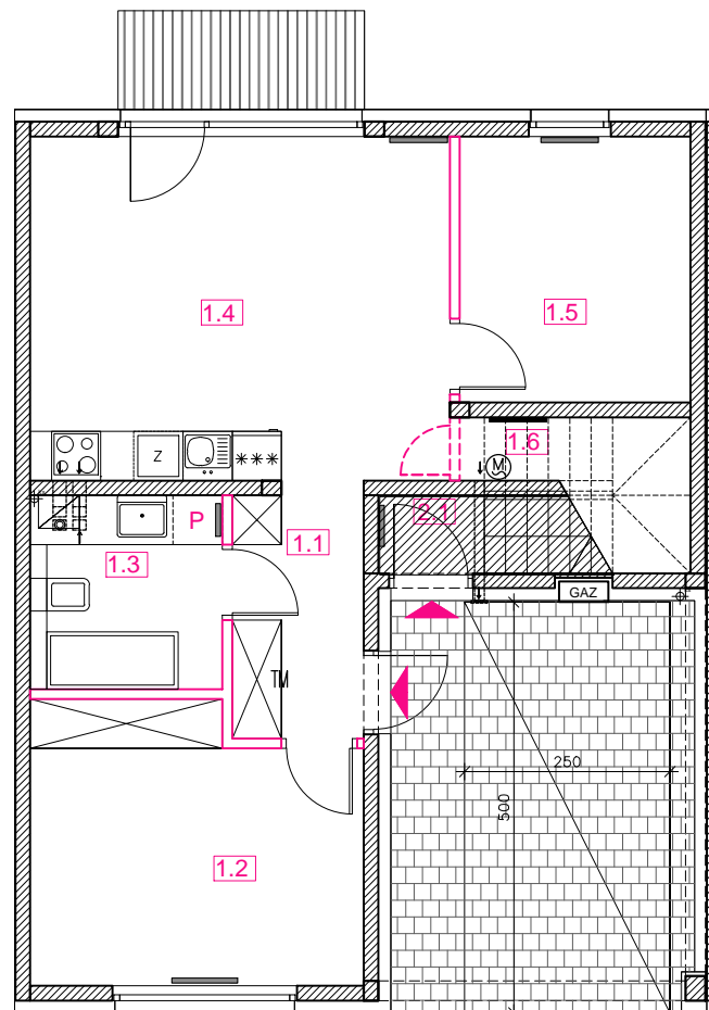
RZUT PARTERU
